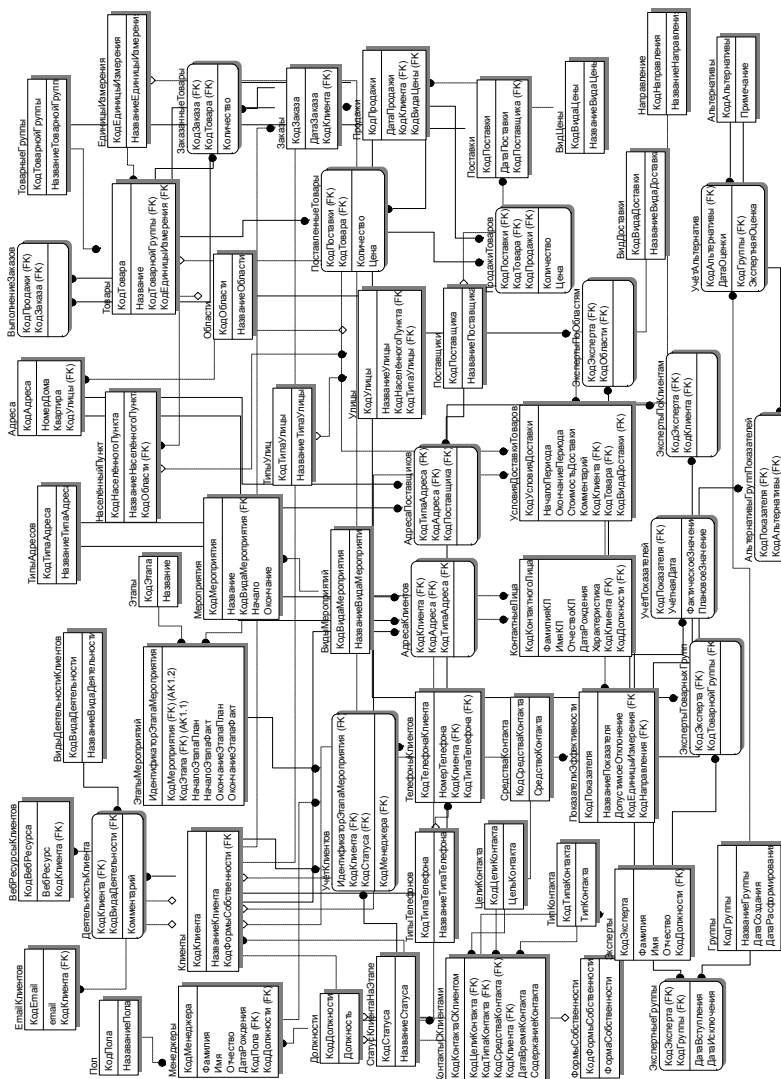
Рис. 1 – Модель даних
