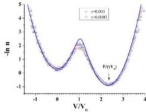
Рис. 3. Залежність функції розподілу часток за швидкостями для різних \gamma при значенні з максимальним D(F) . T' = 0.19 , \nabla - \gamma = 0.003 , \Delta - \gamma = 0.0003 . Суцільною лінією нанесені розрахункові значення виходячи з моделі двух'ямний потенціалу [9]. Функція має мінімуми при V = 0 і V = F/\gamma
